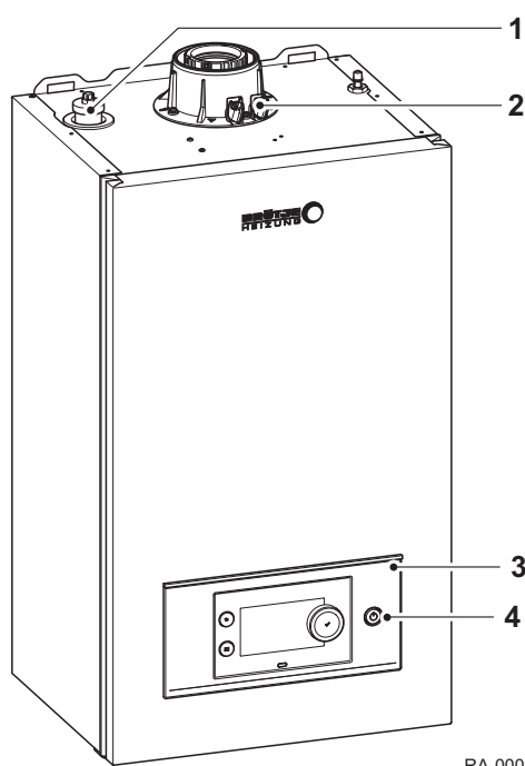
ábra1 Áttekintő rajzWGB-K
