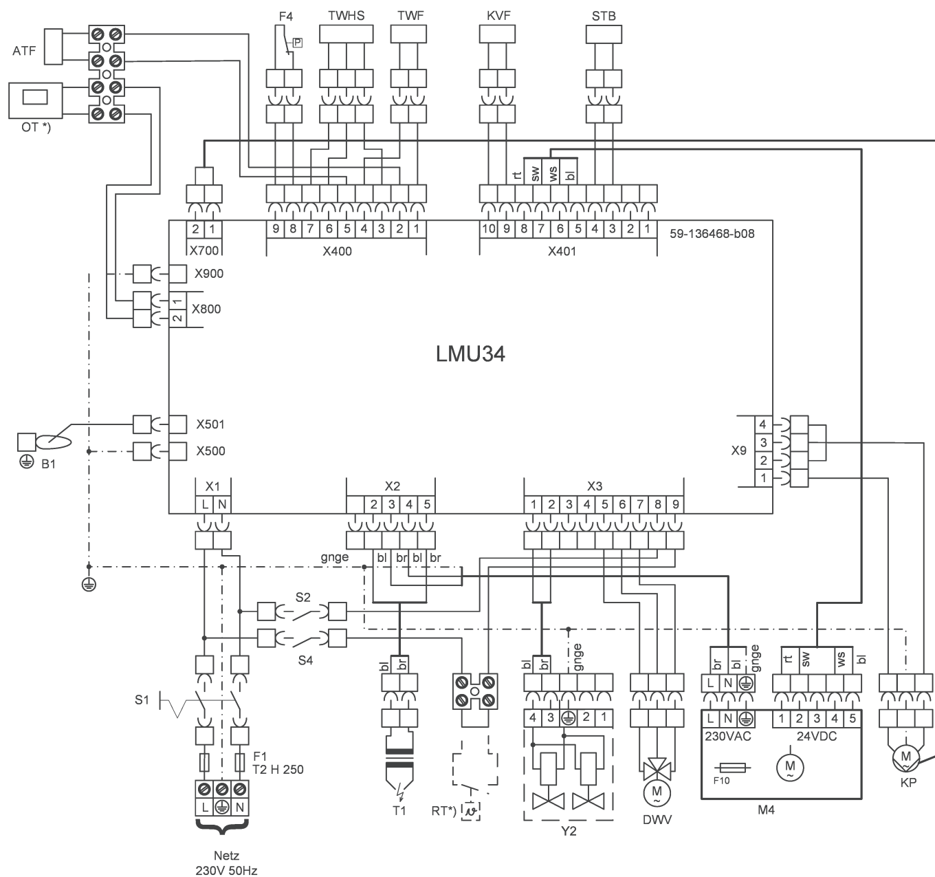
ábra8 Kapcsolási rajzWHBC
