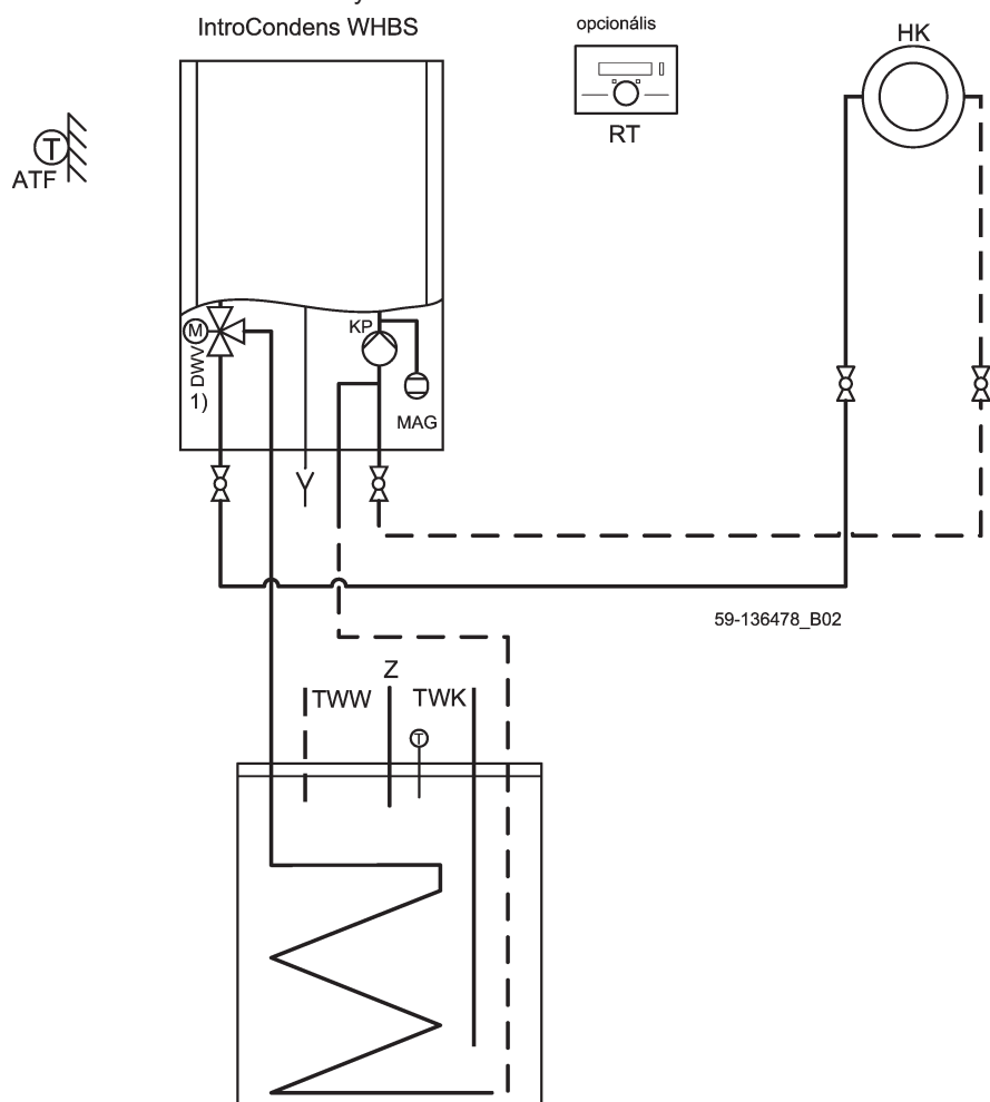
ábra20 Alkalmazási példa: WHBS egy szivattyús fűtési körrel és helyiségtermostáttal, beleértve a tároló hőmérsékletszabályozását
