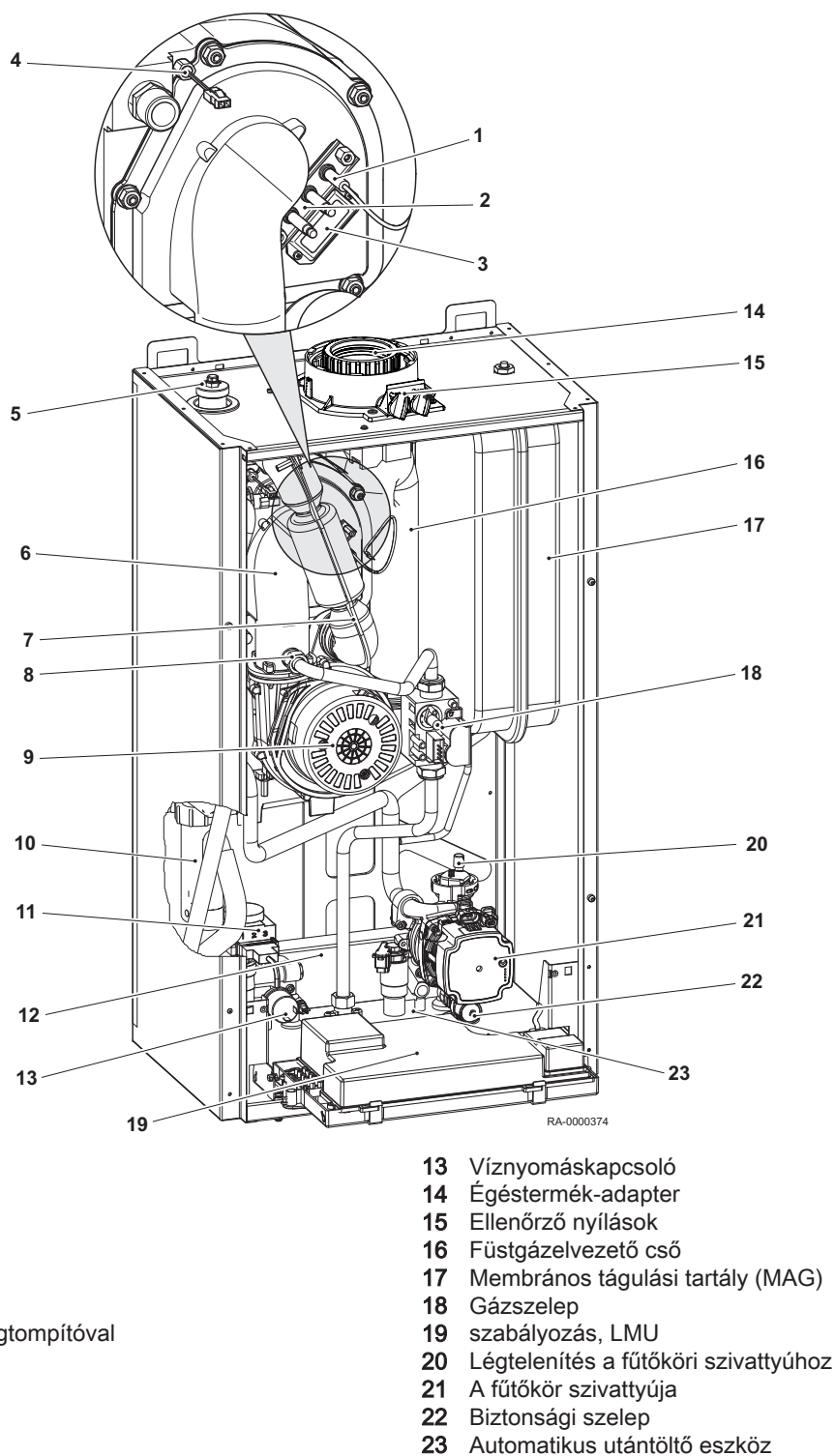
ábra10 Kazánnézet WHBC (homlokfal nélkül ábrázolva)
