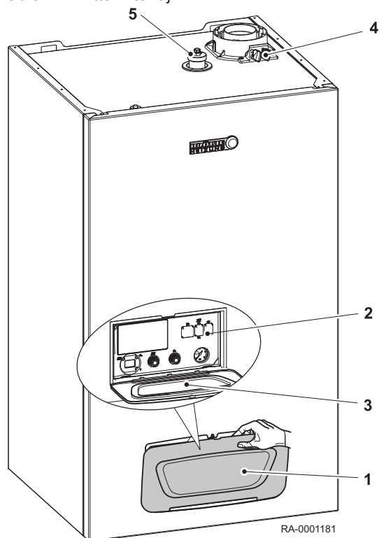
ábra1 Áttekintő rajz WHBK
