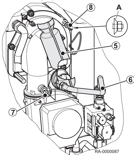
ábra29 Az égőfej leszerelése
