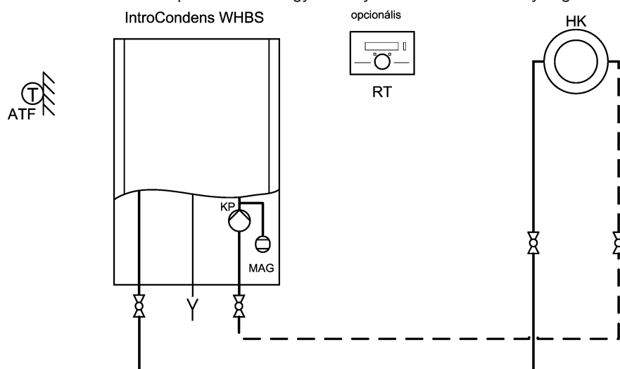
ábra19 Alkalmazási példa: WHBS egy szivattyús fűtési körrel és helyiségtermosztáttal
