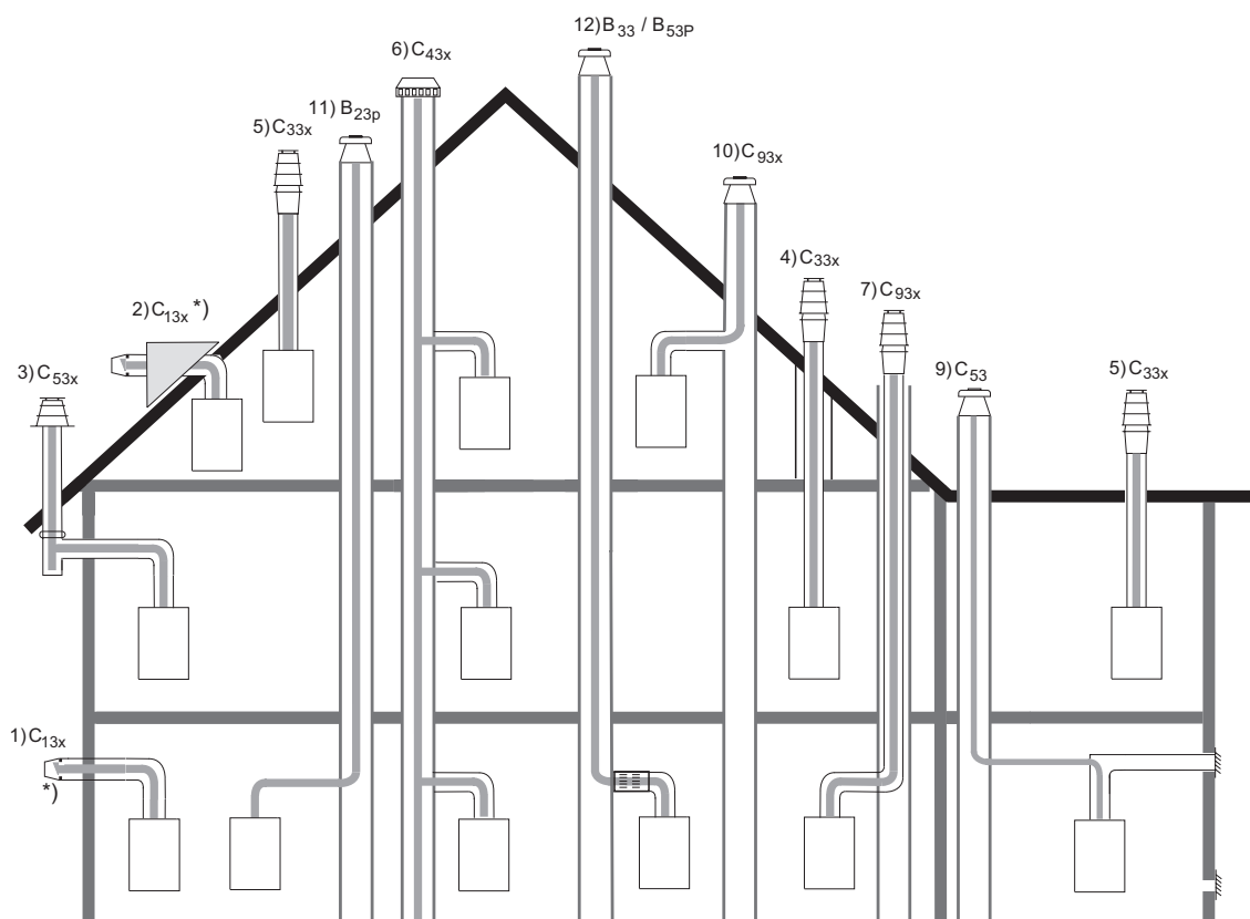
ábra21 Csatlakoztatási lehetőségek a KAS-szal (tartozék)
