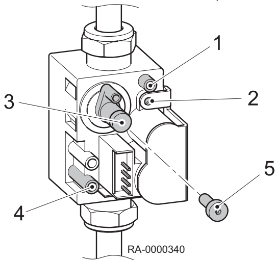
ábra25 Gázszelep (befecskendező nyomás beállítása Torx T15 csavarral)
