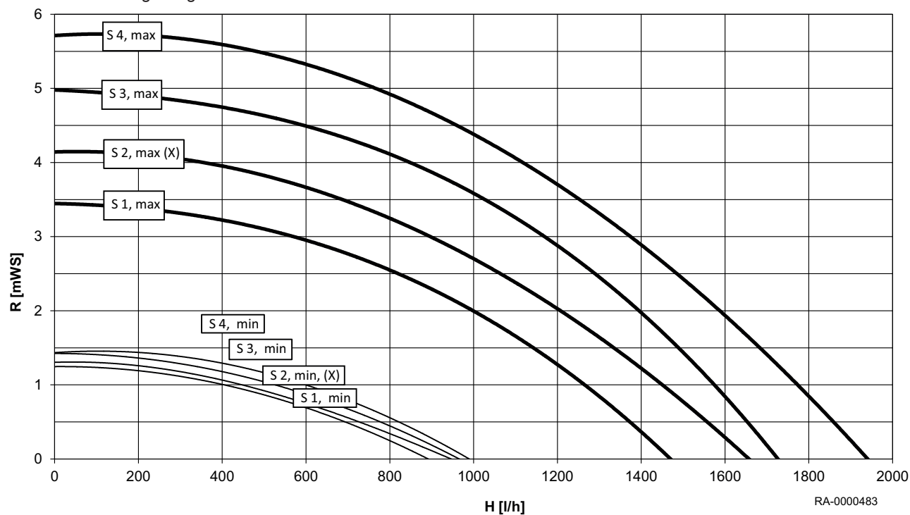
ábra2 Emelőmagasság WHBC28/33
