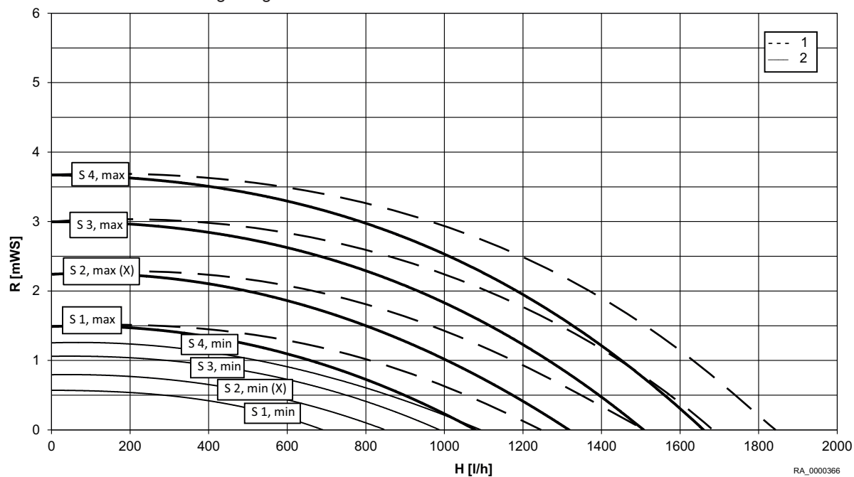
ábra3 Maradó emelőmagasság WHBS 14
