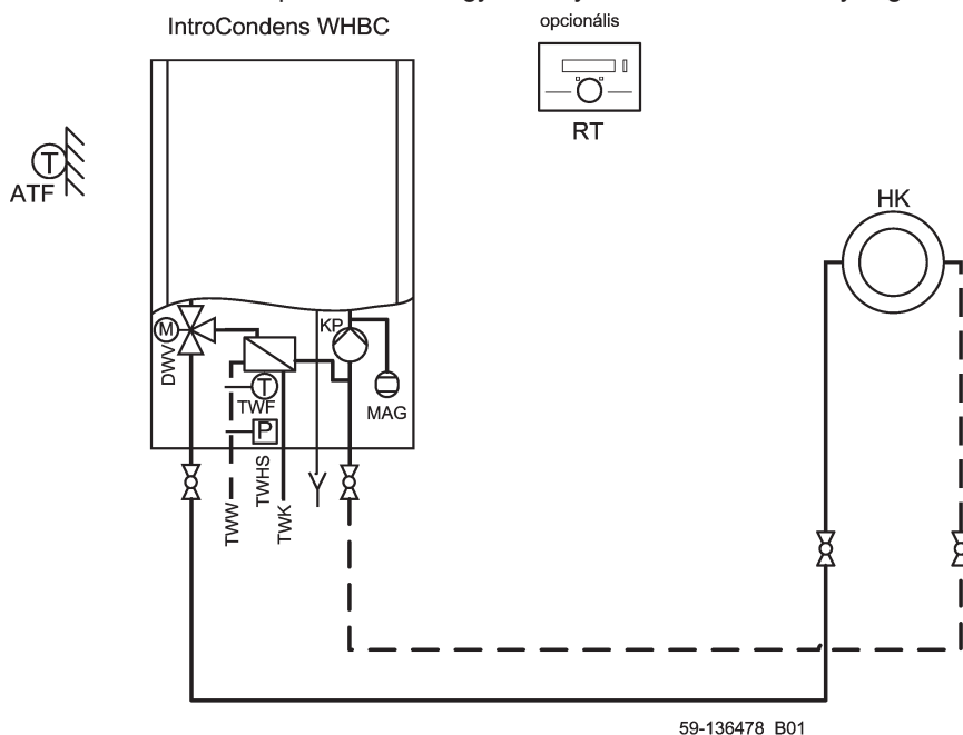
ábra18 Alkalmazási példa: WHBC egy szivattyús fűtési körrel és helyiségtermosztáttal
