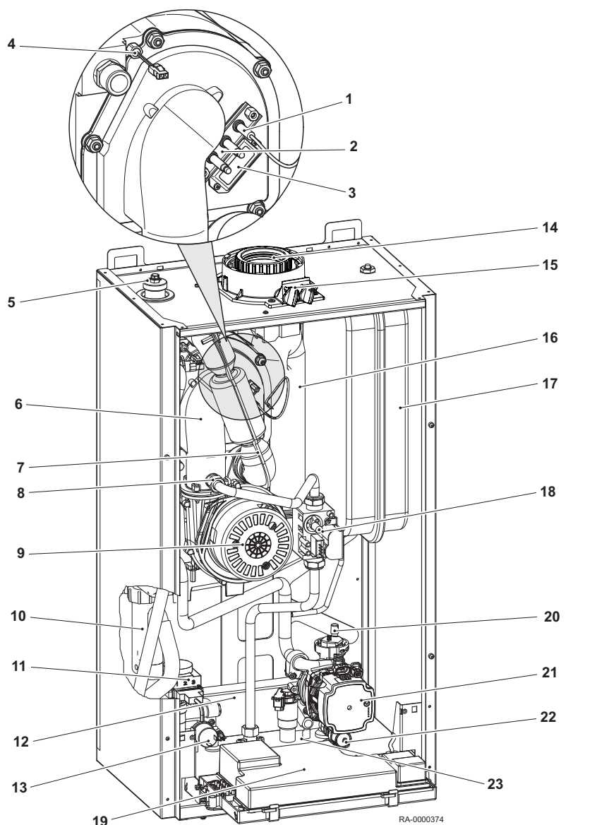
ábra10 Kazánnézet WHBC (homlokfal nélkül ábrázolva)
