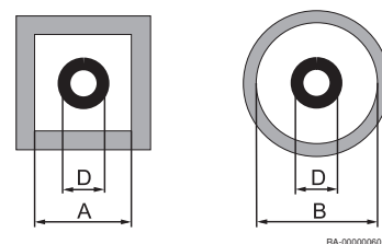
ábra24 Az akna minimális mérete
