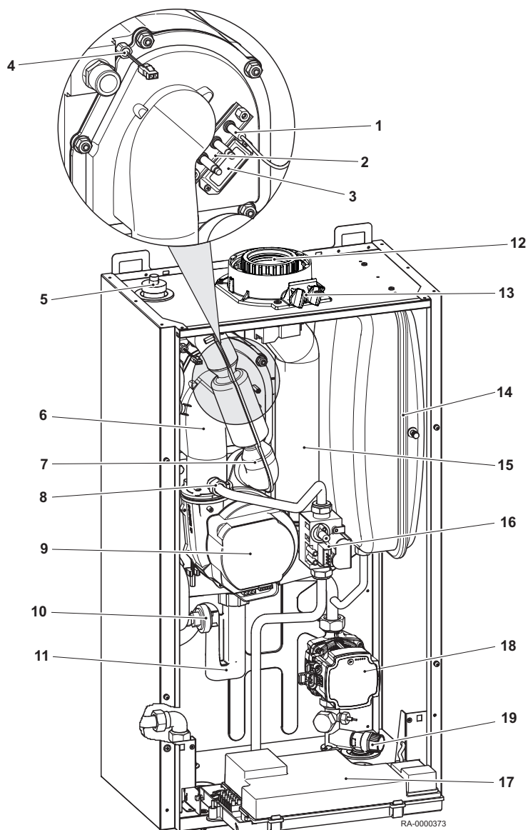
ábra11 Kazánnézet WHBS (homlokfal nélkül ábrázolva)
