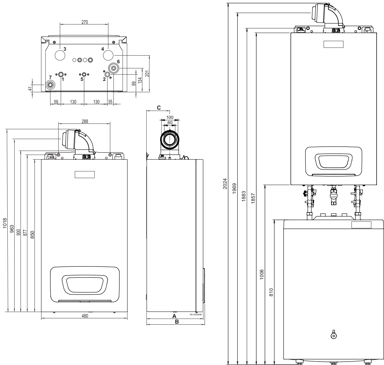
ábra7 Méretek és csatlakozások WHBS
