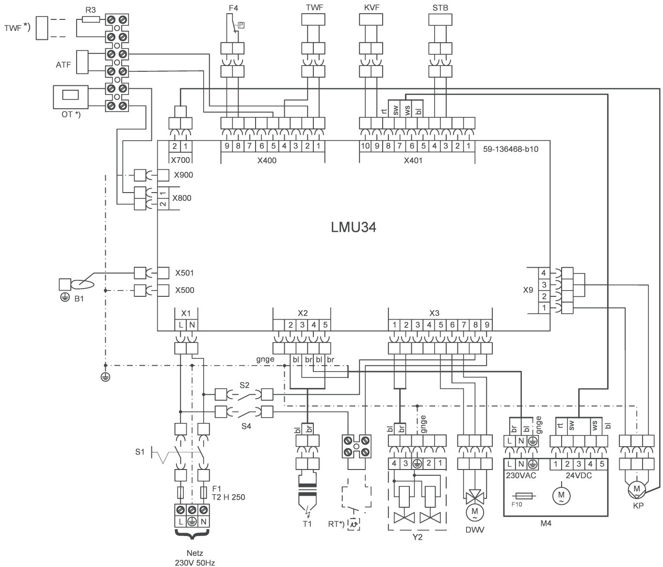
ábra9 Kapcsolási rajzWHBS
