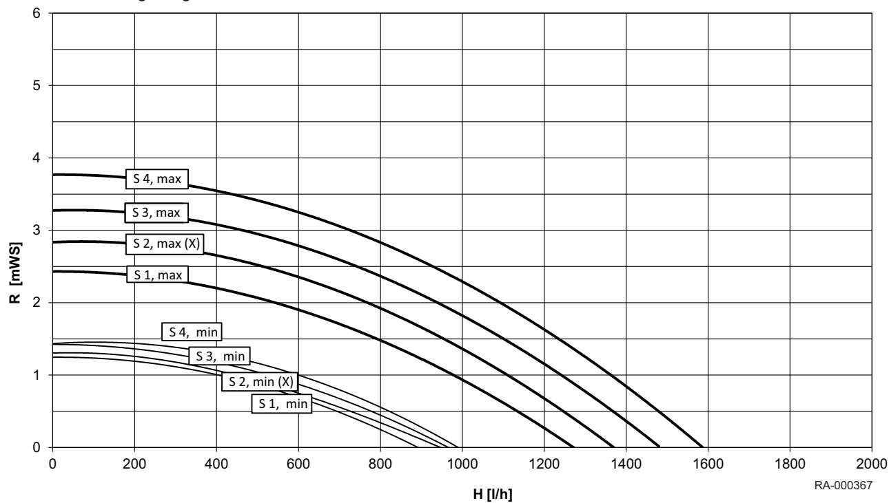
ábra1 Emelőmagasság WHBC22/24
