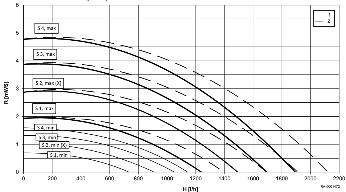
ábra5 Maradó emelőmagasságWHBS 30
