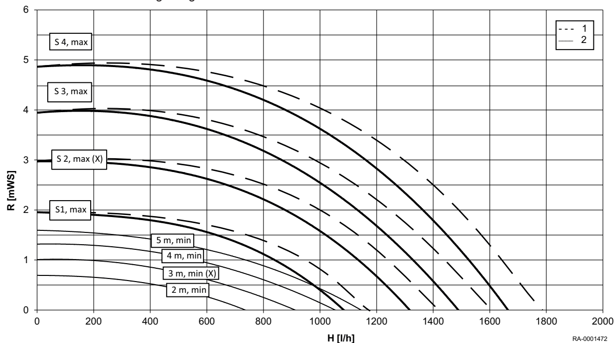
ábra4 Maradó emelőmagasságWHBS 22
