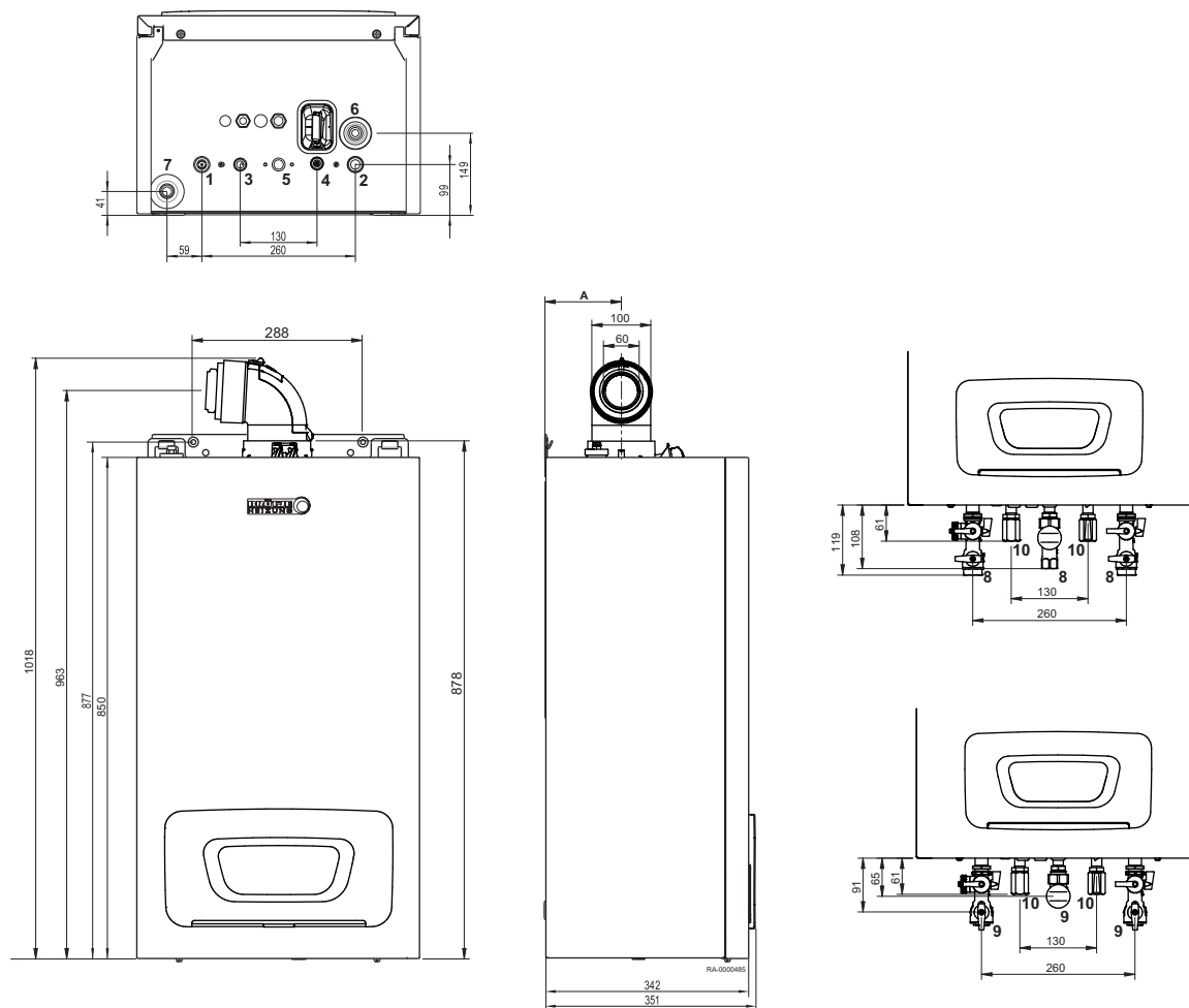
ábra6 Méretek és csatlakozások WHBC
