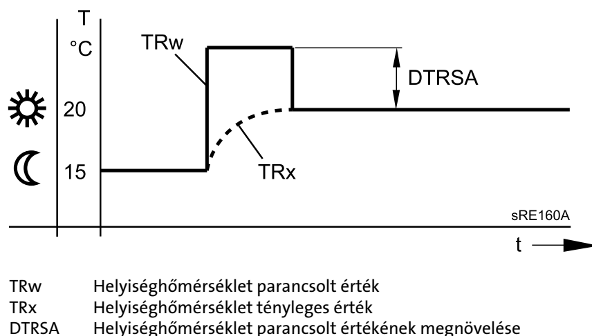
Ábra. 18: Gyors felfűtés
