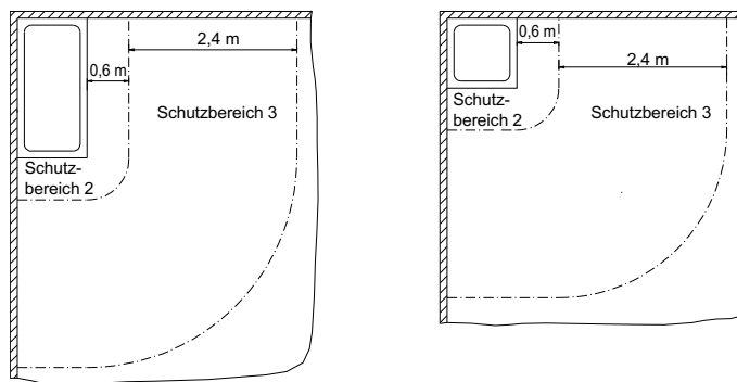
Ábra. 3: A távolságok fürdőszobákban illetve zuhanyozókban.
