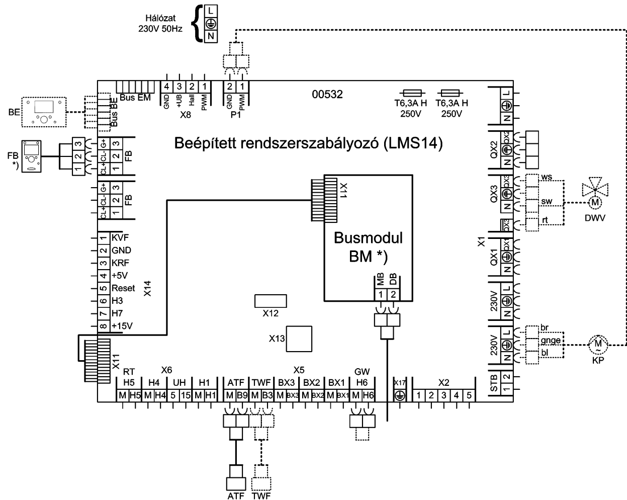
Ábra. 5: Csatlakozási terv
