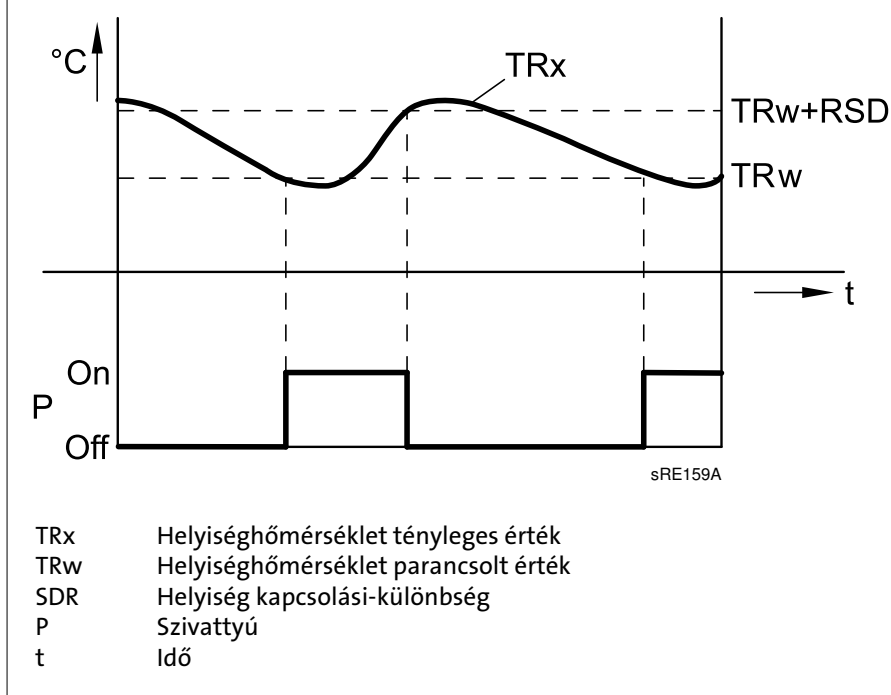
Ábra. 17: Helyiséghőmérséklet-korlátozás
