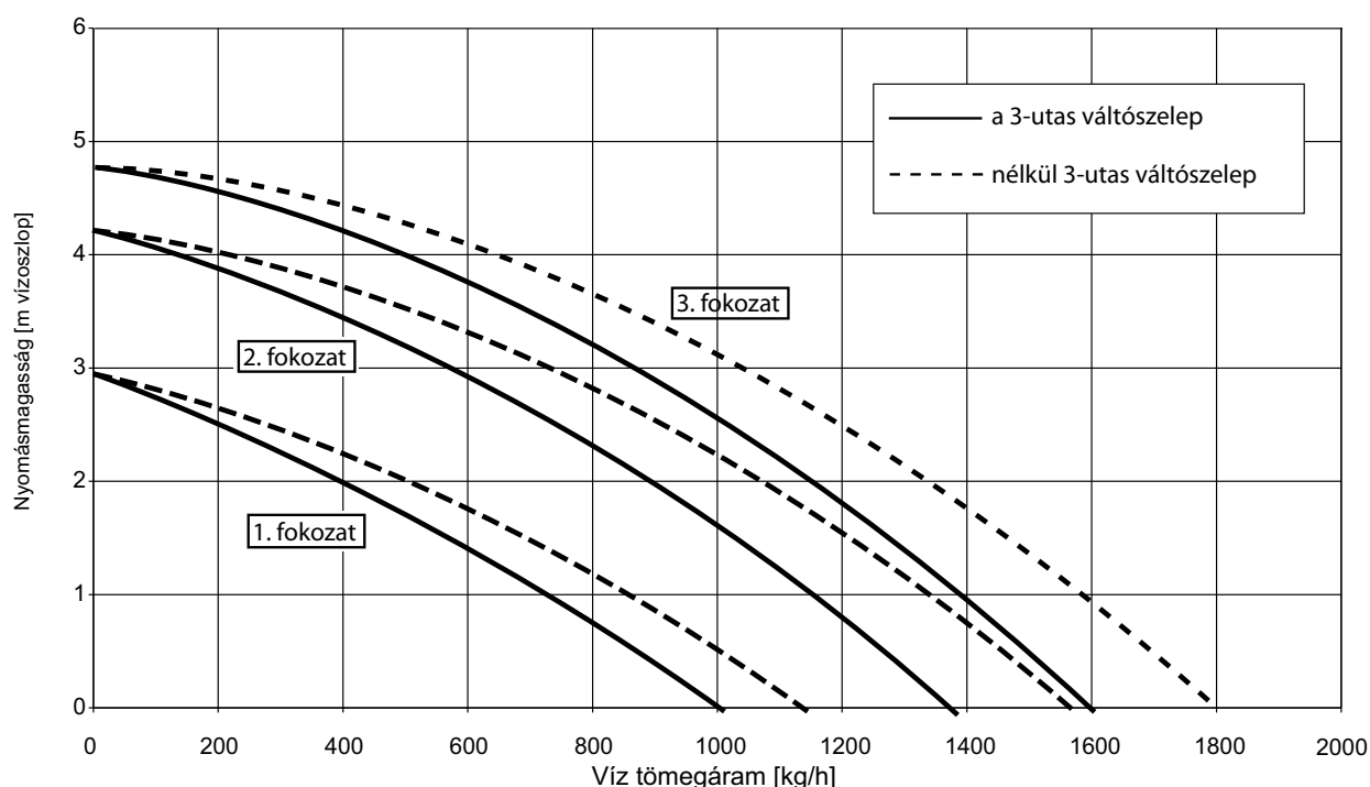
Ábra. 22: Maradék szállítómagasság, WBC 22/24 E
