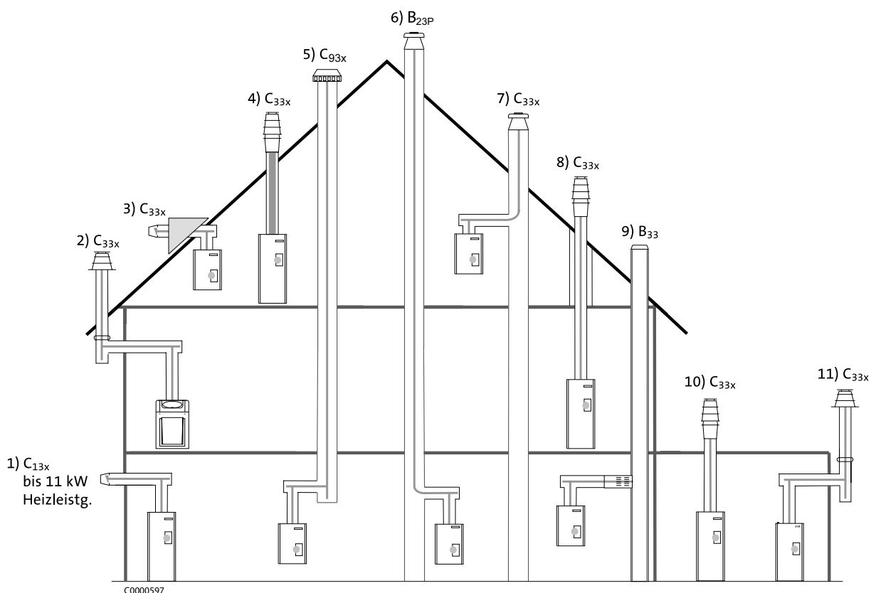
Ábra. 7: Bekötési lehetőségek a KAS -sal (tartozék)
