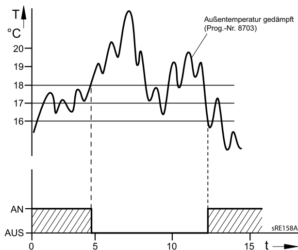
Ábra. 16: Nyári-/téli fűtési határ
