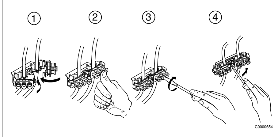
Ábra. 12: Tehermntesítés
