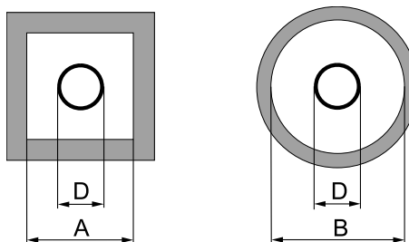
Ábra. 13: A kürtő minimális méretei
