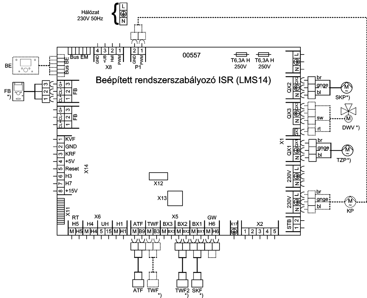
Ábra. 9: Csatlakozási terv
