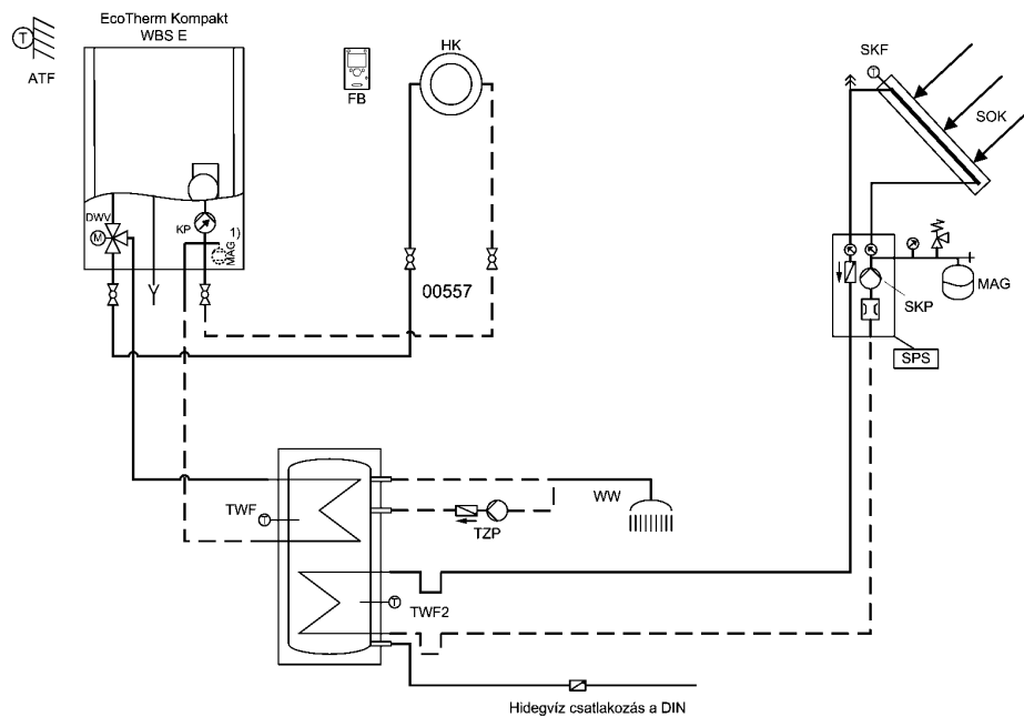
Ábra. 8: Alkalmazási példa: Egy szivattyús fűtési kör szobatermosztáttal és szolártárolóval
