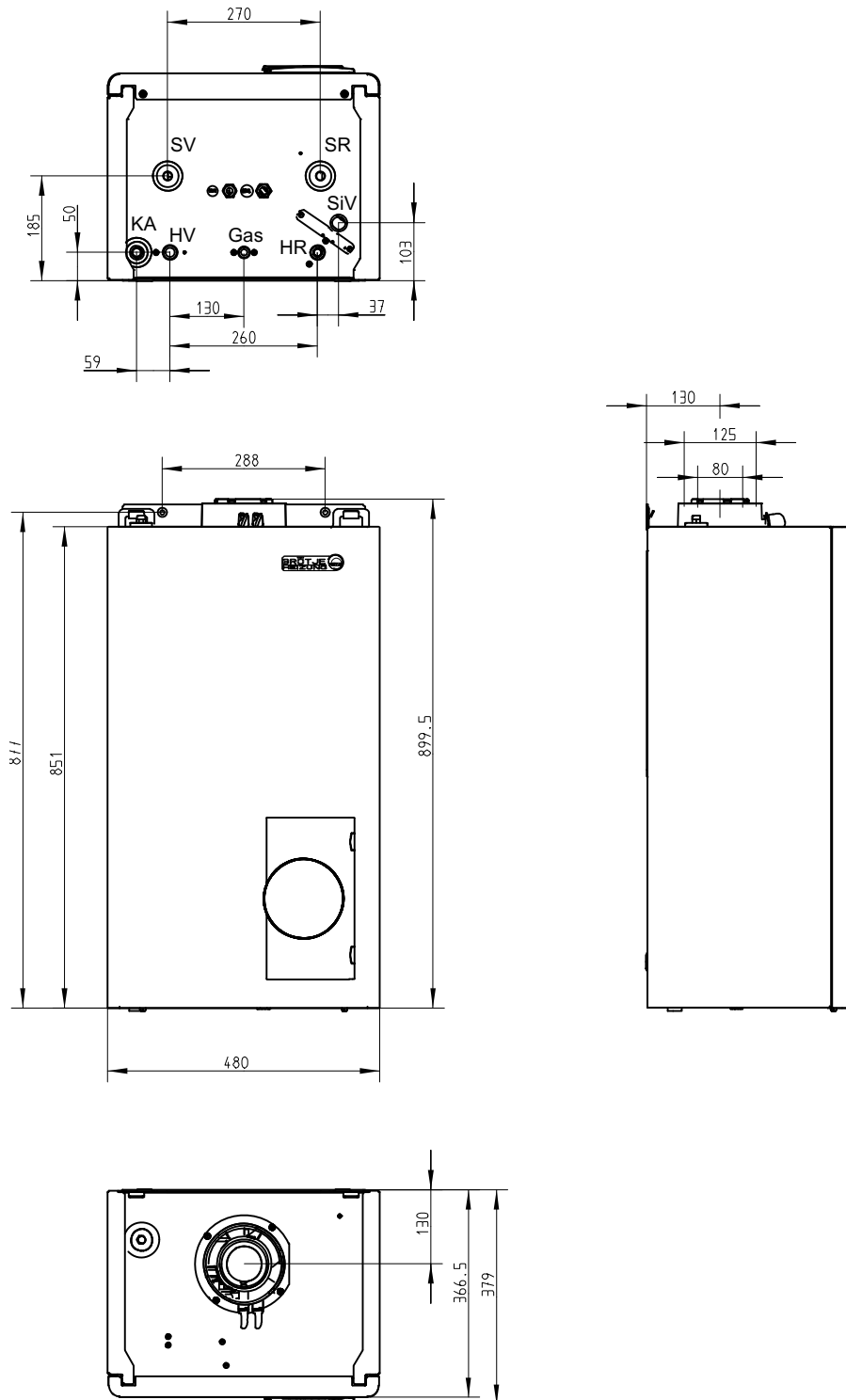
Ábra. 1: Méretek és csatlakozások
