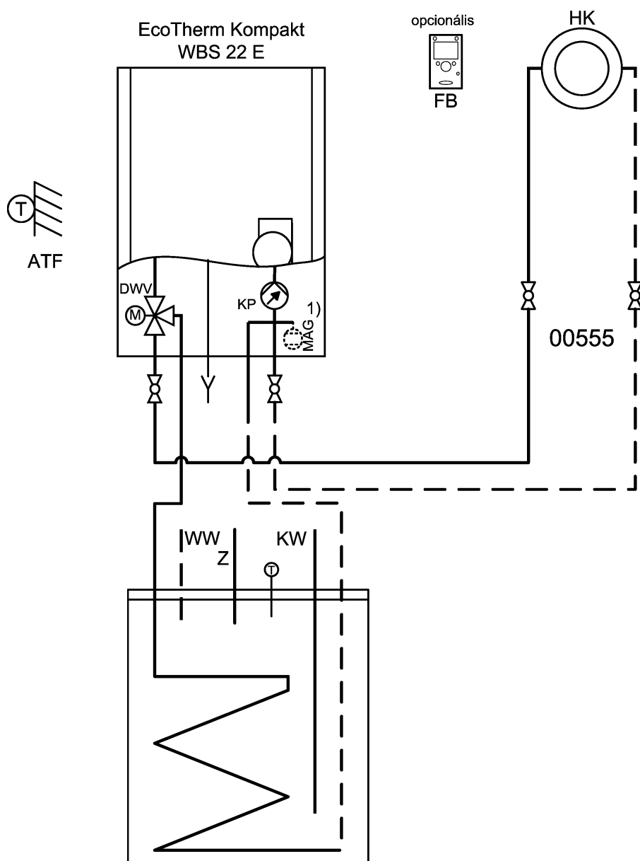
Ábra. 4: Alkalmazási példa: Egy szivattyús fűtési kör szobatermosztáttal, beleértve a tárolóhőmérséklet-szabályozást.
