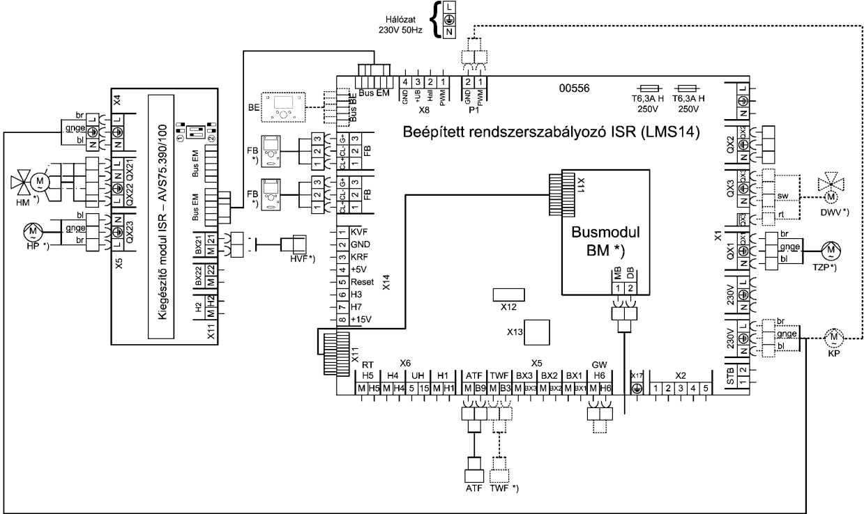
Ábra. 7: Csatlakozási terv
