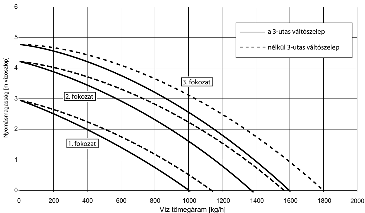
Ábra. 25: Maradék szállítómagasság, WBS 14/22 E
