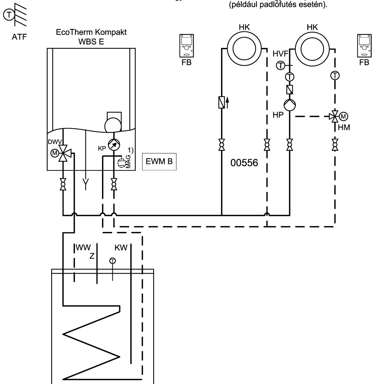
Ábra. 6: Alkalmazási példa: Két szivattyús fűtési kör szobatermosztáttal, beleértve a tárolóhőmérséklet-szabályozást.
