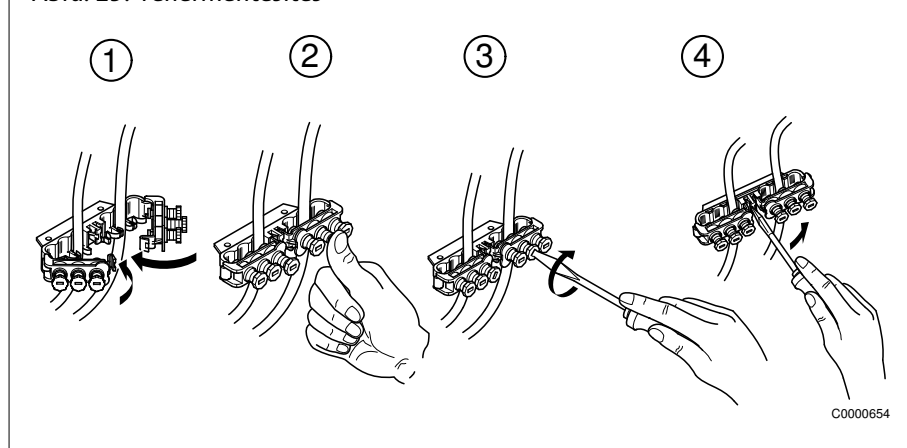
Ábra. 15: Tehermentesítés
