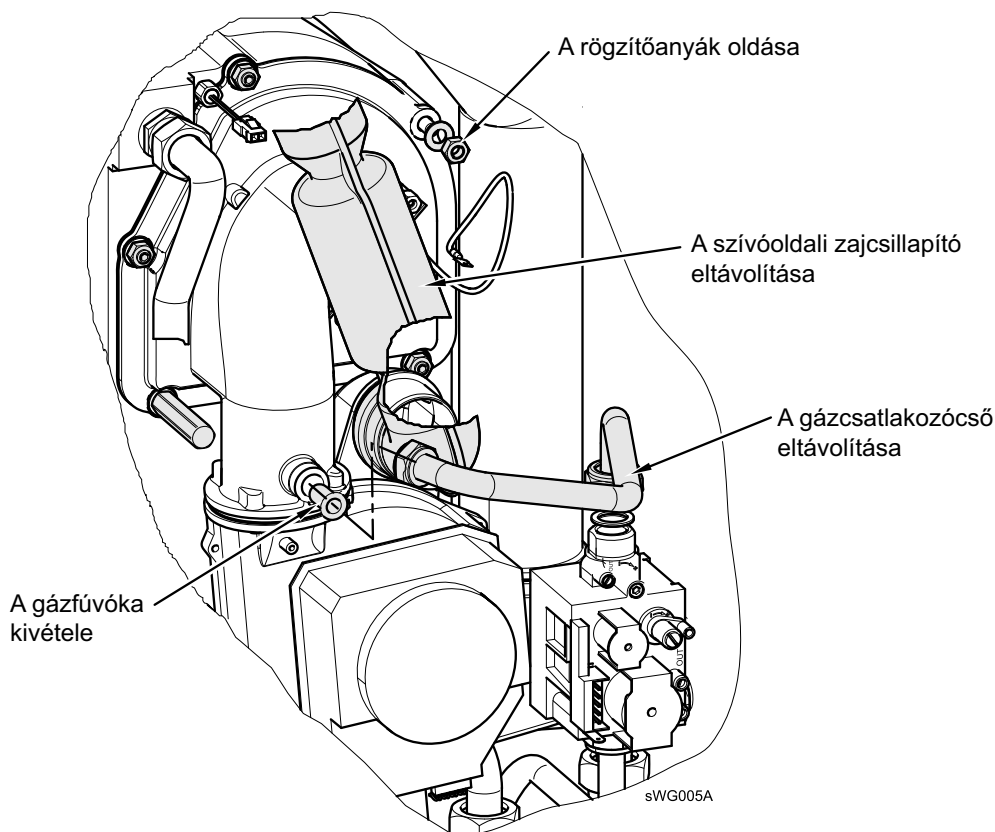
Ábra. 31: A gázégő kiszérése
