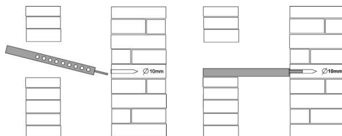
Ábra. 11: A támasztósínek szerelése
