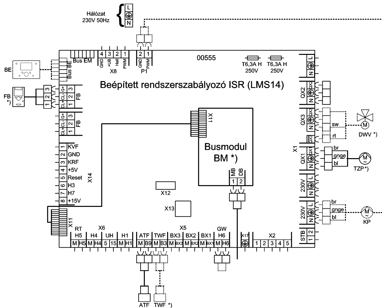
Ábra. 5: Csatlakozási terv
