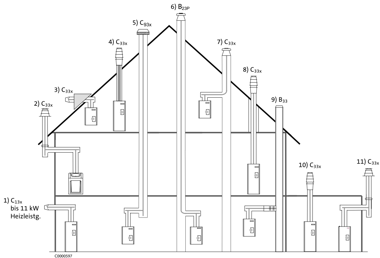
Ábra. 10: Bekötési lehetőségek a KAS -sal (tartozék)
