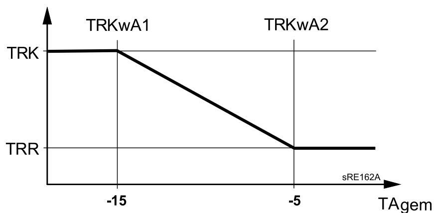
Ábra. 23: Csökk. alapjel emelés
